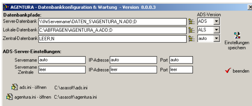
Abb. Agentura-Datenbankkonfiguration mit ADS über File-Ebene
